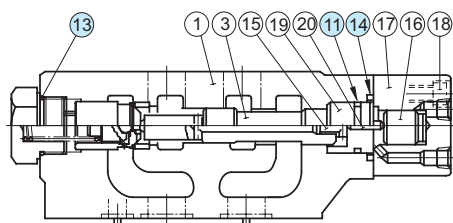
ZPA-32-*-X-30/3090
