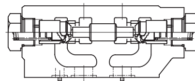
ZPW-32-*-30/3090
