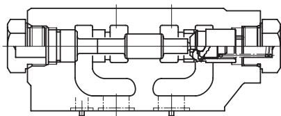
ZPB-32-*-30/3090
