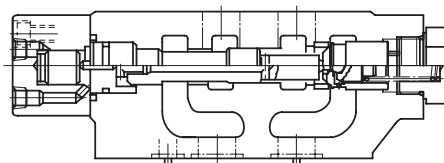
ZPB-32-*-X-30/3090
