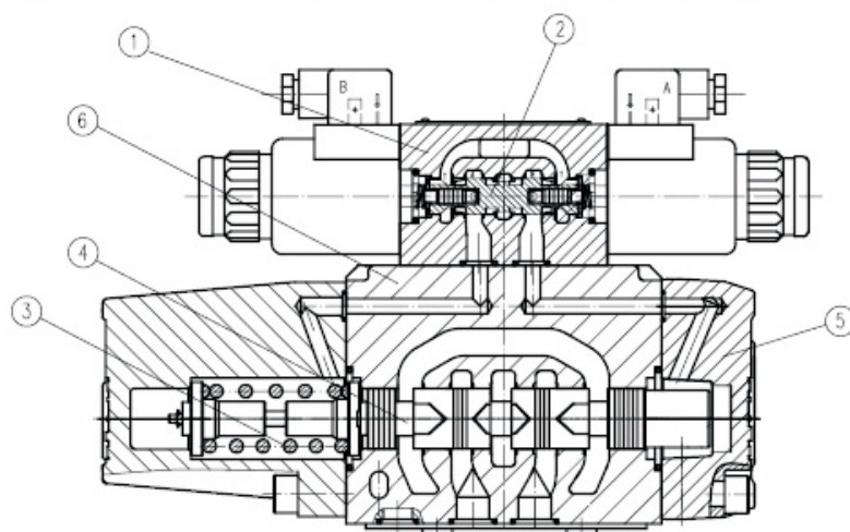
Type HD-4WRZ...-7X/...
