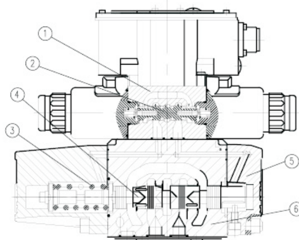
Type HD-4WRZE...-7X/...
