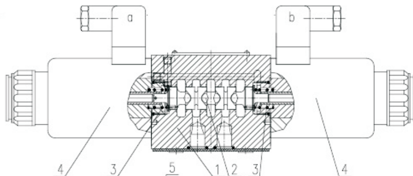
HD-4WRA...-2X/G24K4
