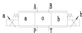
HD-4WRA...A-2X/...
